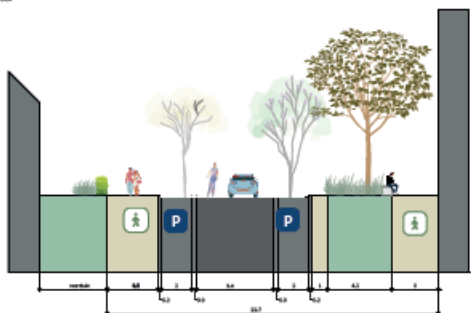
Dwarsprofiel toekomstige situatie
