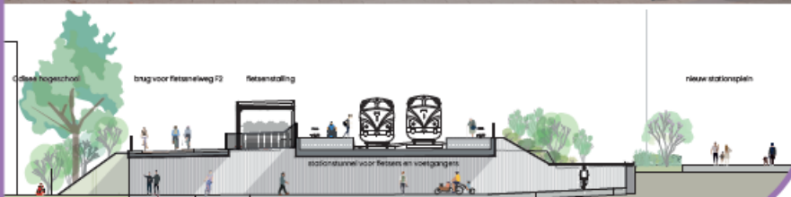
Doorsnede doorheen de toekomstige stationstunnel
